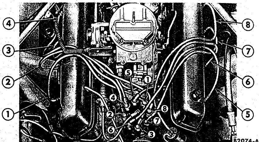
FIG. 34—V-8 Ignition Wiring
